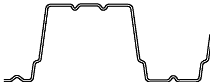
Рисунок 3 — Профили с элементами жесткости на полках и стенках
