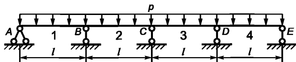
Рисунок 8 — Четырехпролетная неразрезная схема работы профиля
