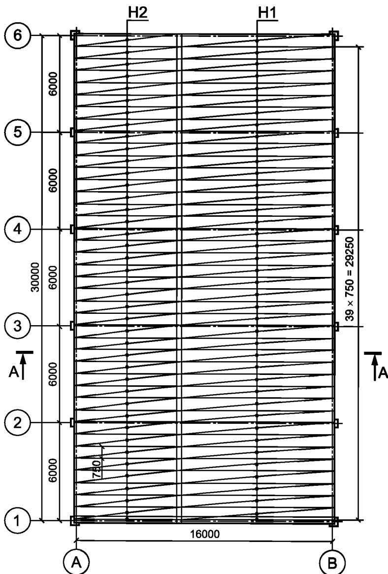
Рисунок А.4 — Схема раскладки профиля
