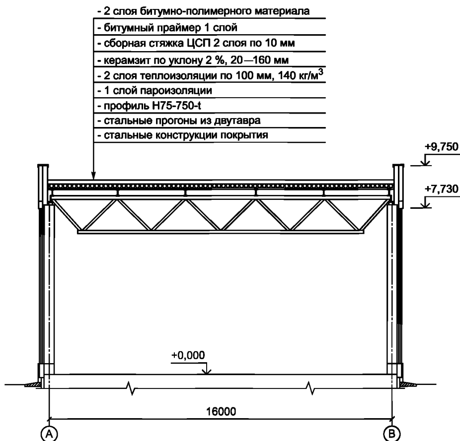
Рисунок А.1 — Поперечный разрез здания спортзала
